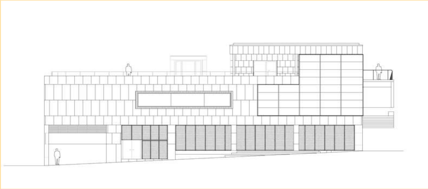
ALZADO RÚA DO PROGRESO
