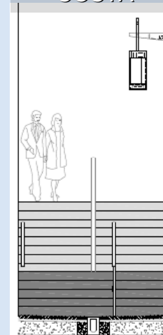
SECCIÓN SUBIDA Á COSTA
